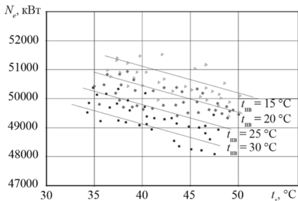
Рис. 2. Мощность МОД в зависимости от температуры наддувочного воздуха t_s при различных температурах воздуха на входе t_{nb} для двигателя 12K98MC-C фирмы «MAN B&W»
