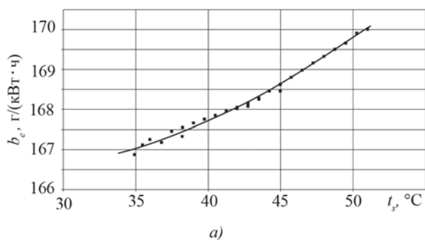
Рис. 3. Удельный расход топлива двигателя b_e в зависимости от температуры наддувочного воздуха t_s при постоянной нагрузке двигателя и различных температурах воздуха на входе t_{nb} :
